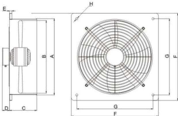
安装尺寸图 Mounting dimensions
